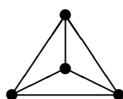
"Tetraeder" m = n = 3
